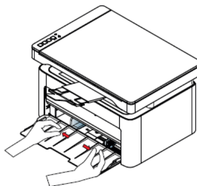
2 Отрегулируйте направляющие
